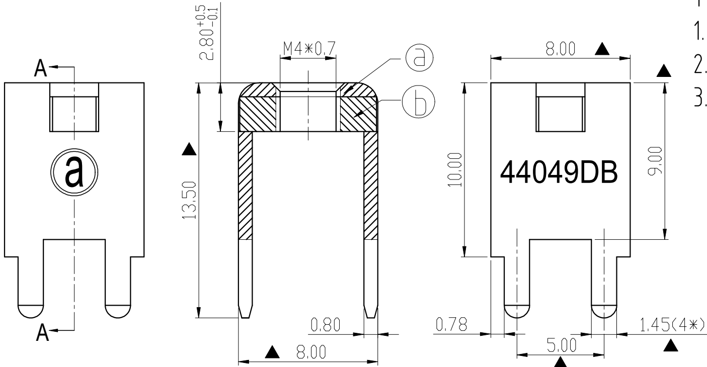
SECTION A-A
