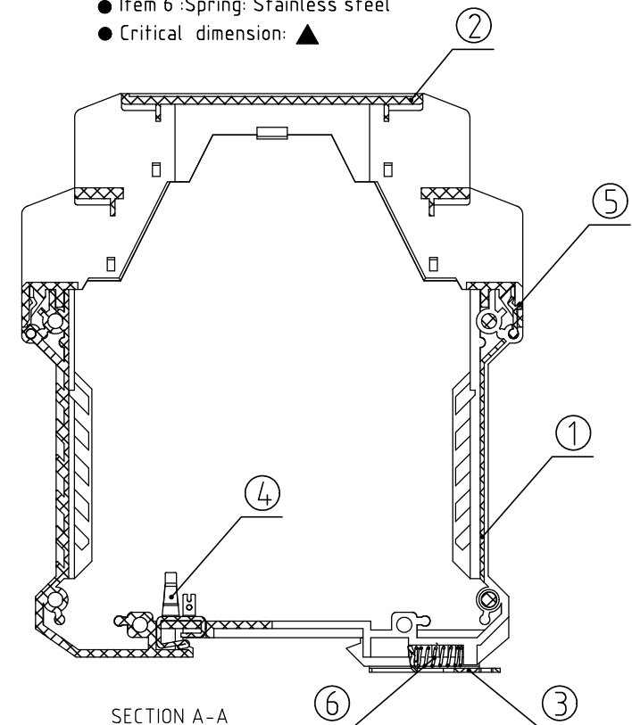
SECTION A-A
